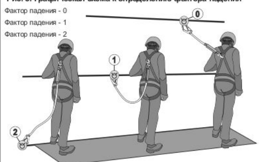
Рис. 8. Графическая схема к определению фактора падения
