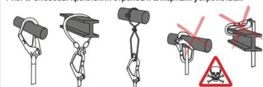
Рис. 6. Способы крепления стропов к анкерным устройствам
