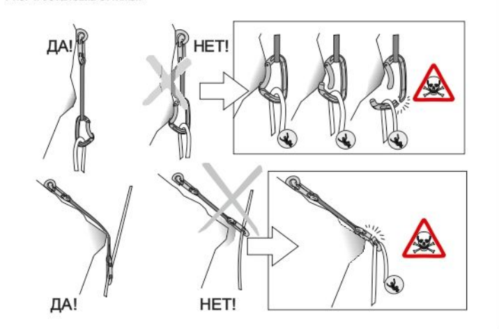
Рис. 4. Установка оттяжек
