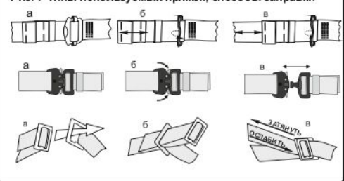
Рис. 7. Типы используемых пряжек, способы заправки
