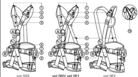
Рис. 1. Общий вид привязей «Профи», расположение и предназначение точек в зависимости от модели
