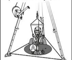
Рис. 16. Способ проведения вертикальной эвакуации
