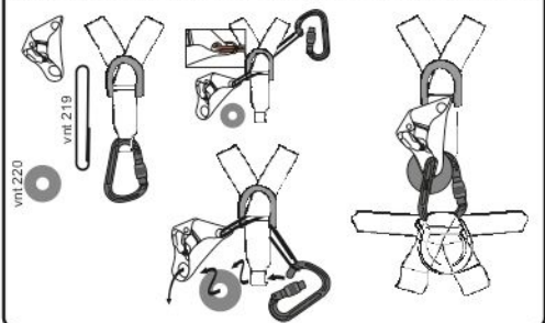
Рис. 13. Соединительно-амортизирующая подсистема
